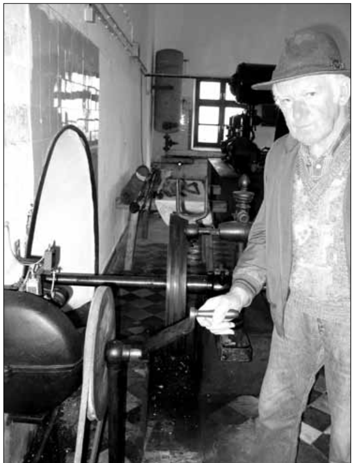
Dank der guten Pflege von Genossenschaftsvorstand Josef Rieder läuft die Turbine noch heute und erzeugt Strom. Foto: Konstanze Kilger
